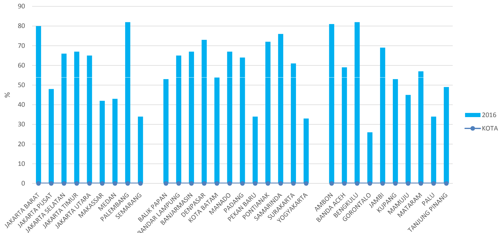
PERSENTASE TINGKAT KETAATAN AMBANG BATAS UJI EMISI KENDARAAN SOLAR 2016
